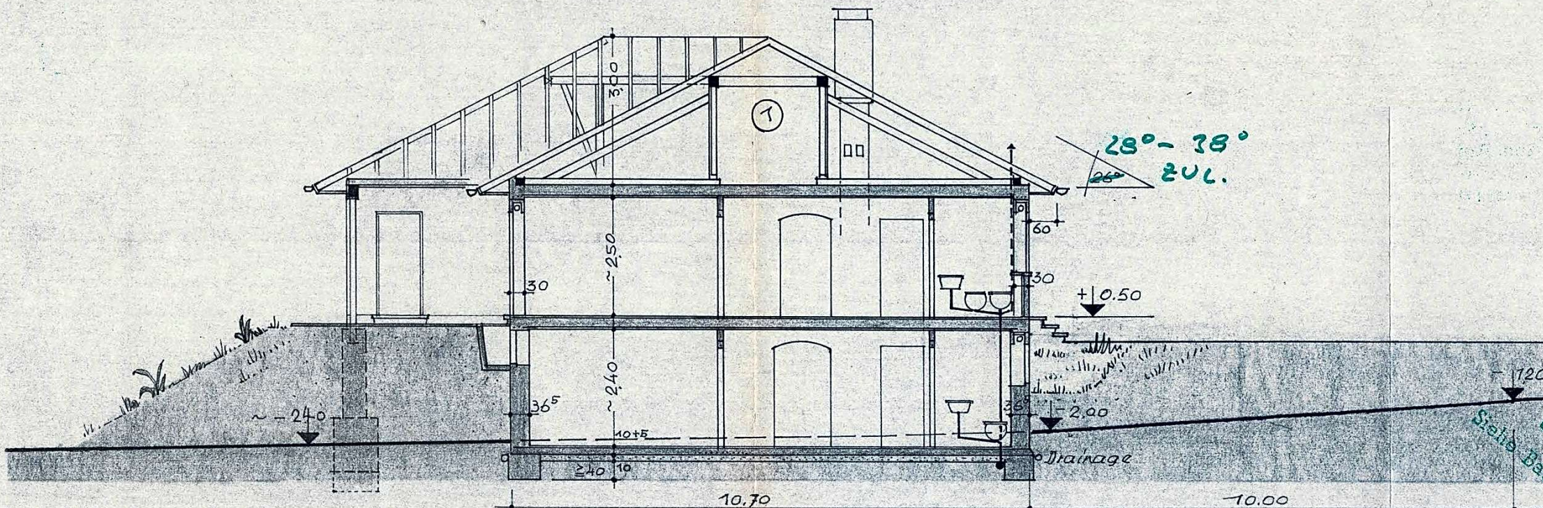
Schnitt A-B
